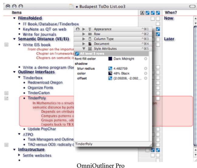
OmniOutliner Pro
