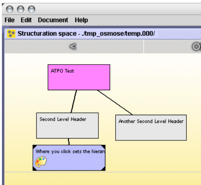
Osmose
