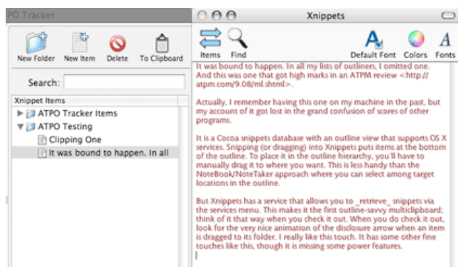
Xnippets
