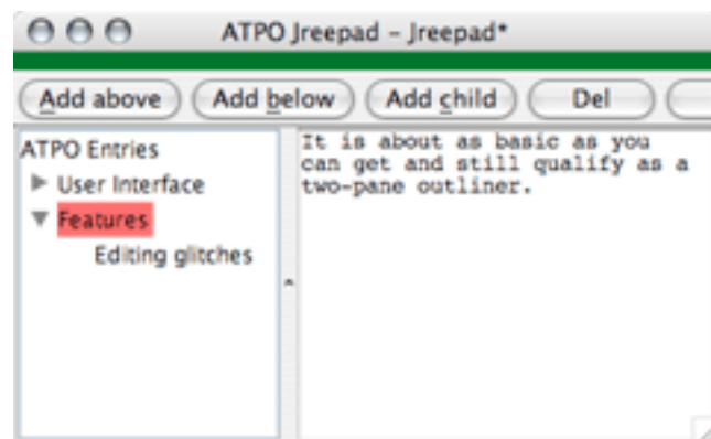
Jreepad
