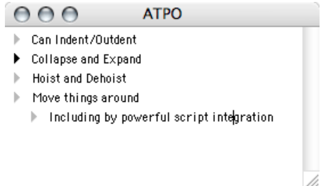
Frontier’s Outliner
