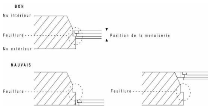
Positionnement des menuiseries nouvelles dans un mur épais ancien.
