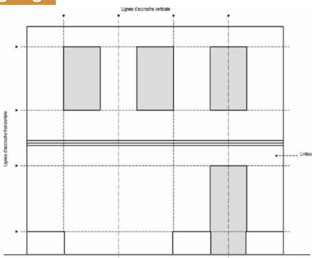
Points d'accroche et lignes de composition des portes cochères ou des portes de garage modernes dans une travée latérale.
