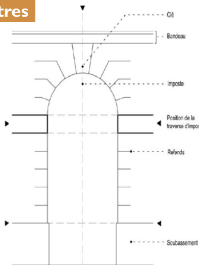
Points d'accroche et lignes de composition des portes d'entrée
